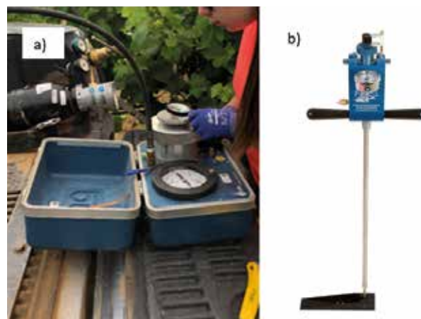
Figura 1. Cámaras de presión tipo Scholander: a) medida de potencial hídrico con cámara alimentada con bombona de gas que proporciona la presión a aplicar, b) cámara sin bombona de gas, la presión es proporcionada por un pistón accionado manualmente.
