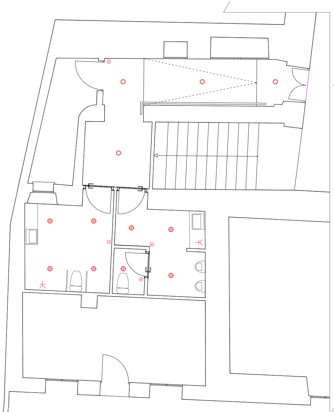
Electricidad e iluminación en baños
